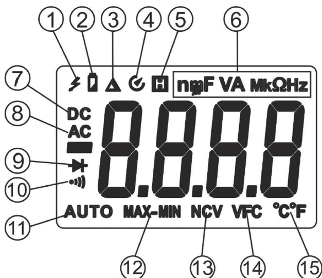
Рис. 2 Дисплей, вид 1
