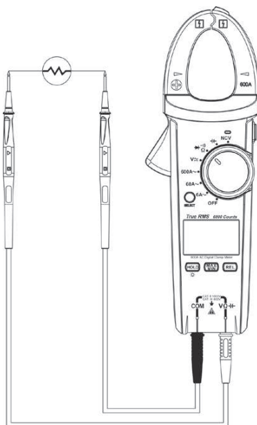
Рис. 10 Проверка диода
