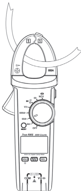
Рис. 4 Измерение силы переменного тока
