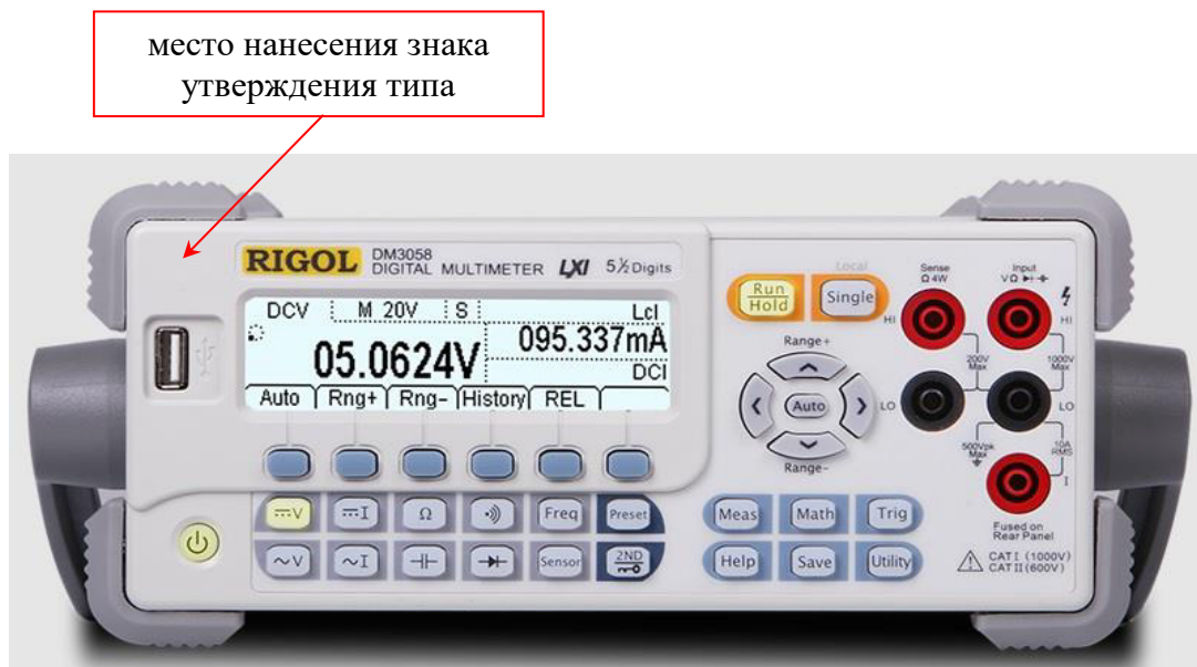
Рисунок 1 – Передняя панель Rigol DM3058
