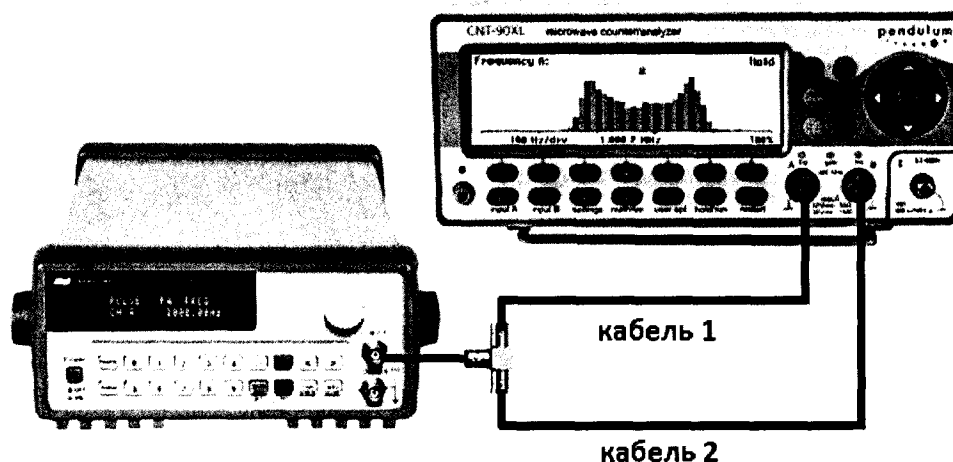
Рисунок 1 – Определение разницы задержки в измерительных кабелях
