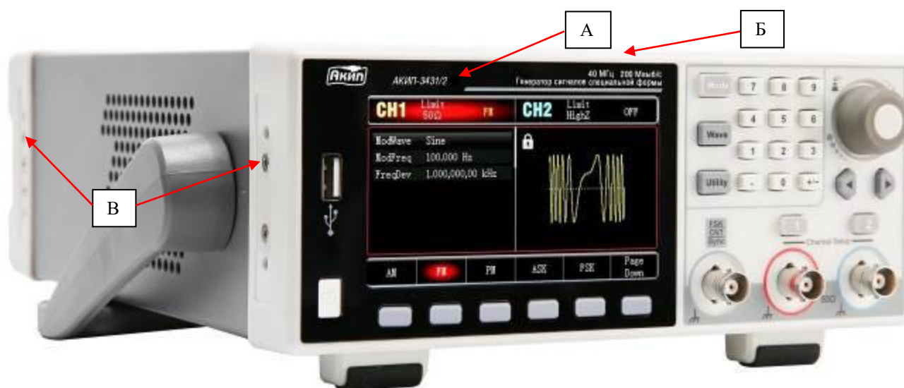
Рисунок 1 – Внешний вид передней панели генератора АКПП-3431 с местами нанесения знака утверждения типа (А), знака поверки (Б) и пломбировки от несанкционированного доступа (В)
